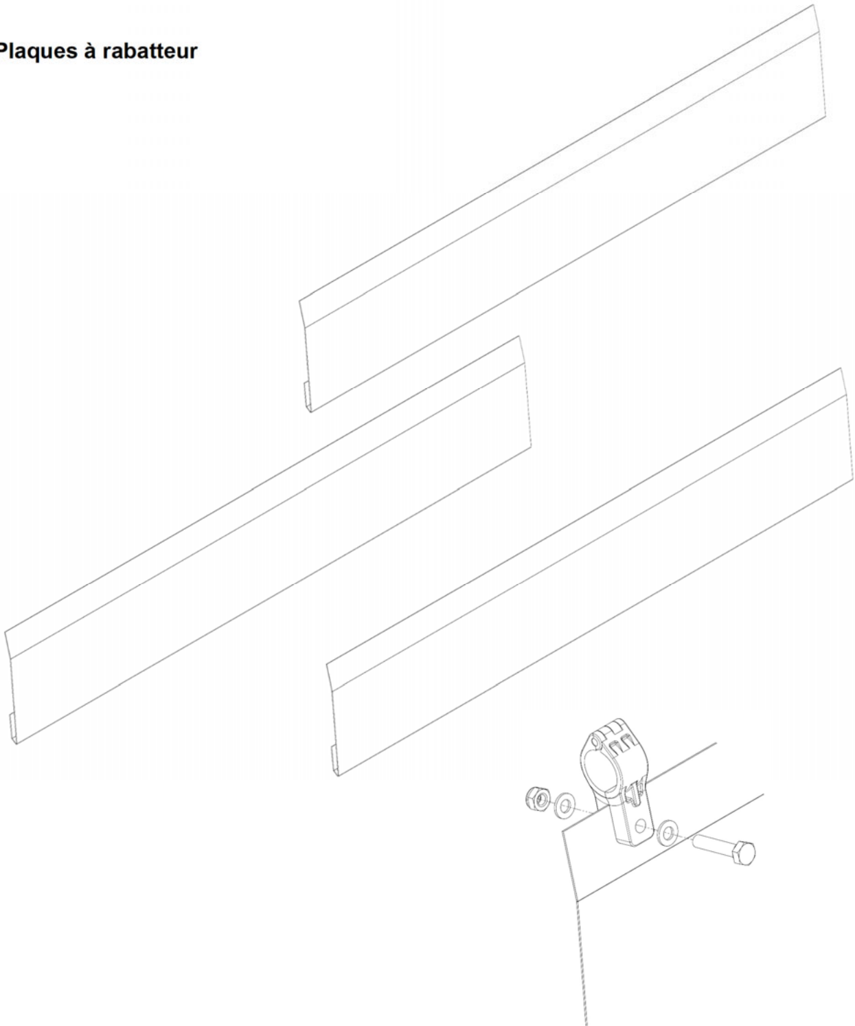
Fixation à rabatteur avec griffes en plastique
