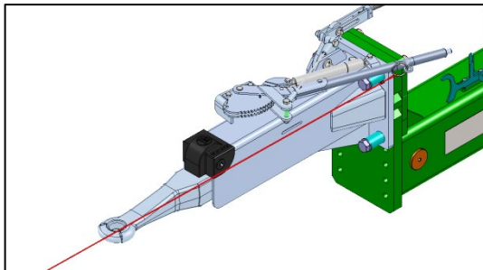
SWW460 - Auflaufkopf.
