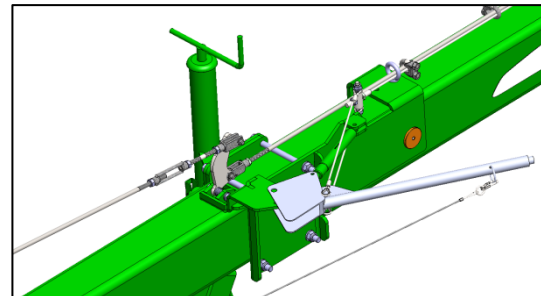
SWW450 - Übertragungseinrichtung – Zugstange zwischen dem Abtriebshebel des Auflaufkopfes und dem Übersetzungshebel.
