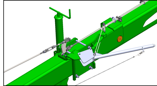
SWW450 - Abreißseil – Anschlagpunkt an Handbremshebel.
