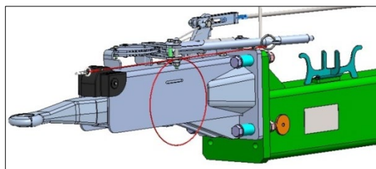
Einstellhöhe 590 mm SWW460
