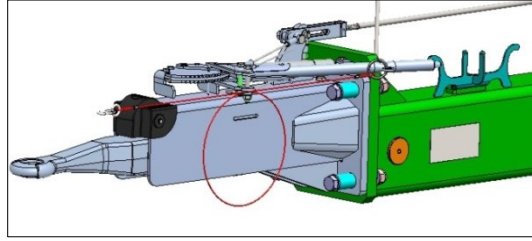
Einstellhöhe 535 mm SWW460
