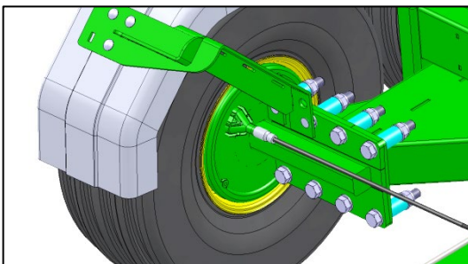
SWW460 - Übertragungseinrichtung – Verbindung zwischen der Ausgleichswaage und den Radbremsen mittels Seilzug
