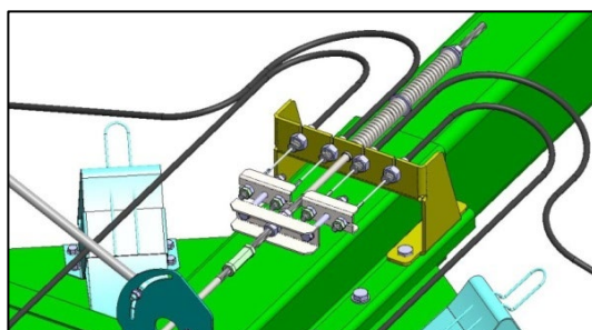
SWW450 - Übertragungseinrichtung – Verteilung der Bewegung der Zugöse im Auflaufkopf auf die 4 Radbremsen mittels der Ausgleichswaage.
