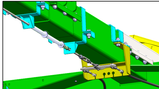
SWW450-HM / SWW460-HM - Übertragungseinrichtung – Zugstange zur Ausgleichswaage mit Lösefederpaket.
