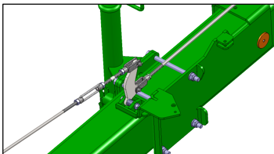
SWW460 - Übertragungseinrichtung – Übersetzungshebel.
