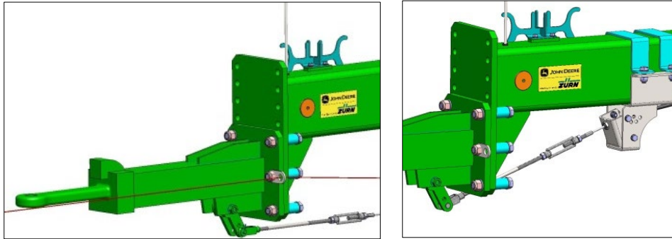
Einstellhöhe 535 mm
