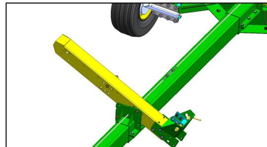
SWW450 - Übertragungseinrichtung – Verbindung zwischen Übersetzungshebel und Achstandem mittels Zugstange mit Spannschloßmutter.
