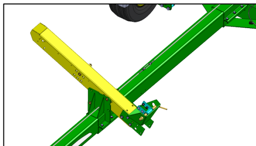
SWW460 - Übertragungseinrichtung – Verbindung zwischen Übersetzungshebel und Achsstandem mittels Zugstange mit Spanschloßmutter.
