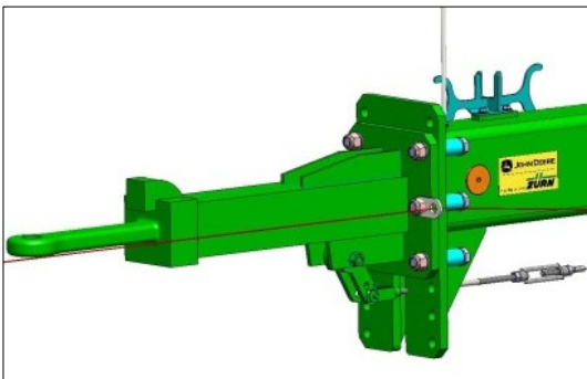
Einstellhöhe 700 mm
