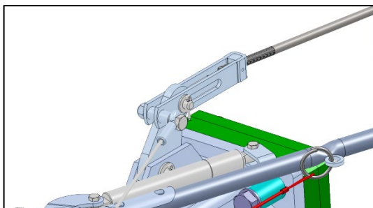
SWW460 - Übertragungseinrichtung – Kulisse zwischen dem Abtriebshebel des Auflaufkopfes und der Zugstange.
