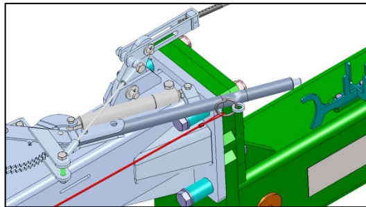
SWW460 - Abreißseil – Anschlagpunkt an Handbremshebel.
