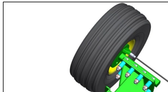
SWW450 - Übertragungseinrichtung – Verbindung zwischen der Ausgleichswaage und den Radbremsen mittels Seilzug
