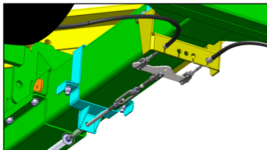
SWW450-HM / SWW460-HM - Übertragungseinrichtung – Zugstange zur Ausgleichswaage mit Spannschloßmutter und Seilzüge zu den Radbremsen.
