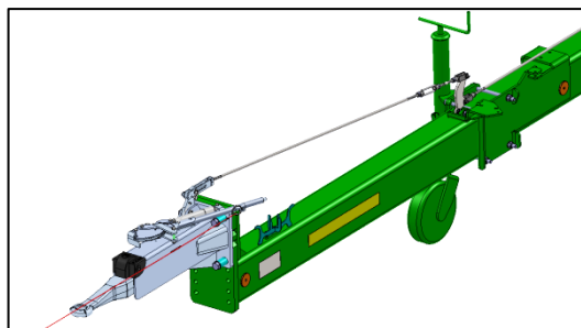
SWW460 - Übertragungseinrichtung – Zugstange zwischen dem Abtriebshebel des Auflaufkopfes und dem Übersetzungshebel.
