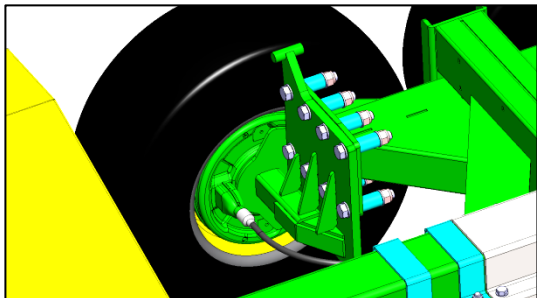
SWW450-HM / SWW460-HM - Übertragungseinrichtung – Seilzug zur Radbremse links vorn.
