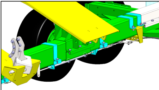
SWW450-HM / SWW460-HM - Übertragungseinrichtung – Zugstange zwischen dem Übersetzungshebel und der Ausgleichswaage vor dem Achstandem.
