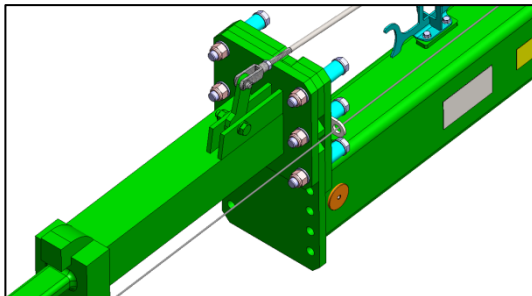
SWW450 - Abreißseil – Führungsblech hinter dem Auflaufkopf.
