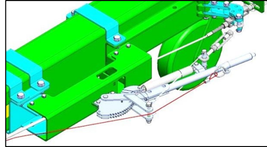
SWW450-HM / SWW460-HM - Abreißseil – Anschlagpunkt an Handbremshebel.
