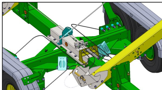
SWW460 - Übertragungseinrichtung – Übertragungseinrichtung – Verteilung der Bewegung der Zugöse im Auflaufkopf auf die 4 Radbremsen mittels der Ausgleichswaage.
