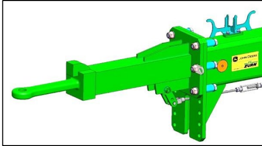
SWW450-HM / SWW460-HM - Auflaufkopf.
