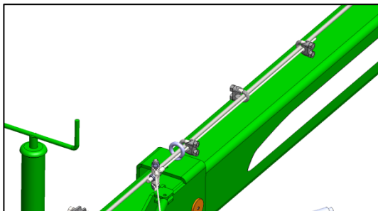
SWW450 - Übertragungseinrichtung – Verbindung der Seile des Handbremshebels mit der Zugstange zwischen Übersetzungshebel und Achstandem.
