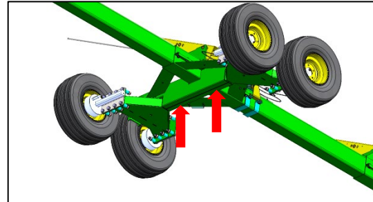
Unterstützung der Achse an den dafür vorgesehenen Punkten
