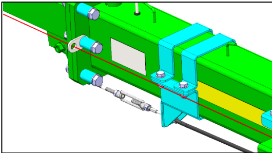
SWW450-HM / SWW460-HM - Abreißseil – Führungsblech hinter dem Auflaufkopf.
