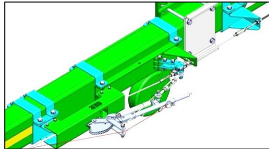
SWW450-HM / SWW460-HM – Übertragungseinrichtung – Seilzug und Spannschloßmutter zwischen dem Handbremshebel und dem Übersetzungshebel.
