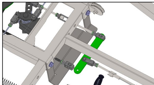
Rechten Bremszug aus der Ausgleichswaage entfernen und mehrmals kräftig nach vorne ziehen.
