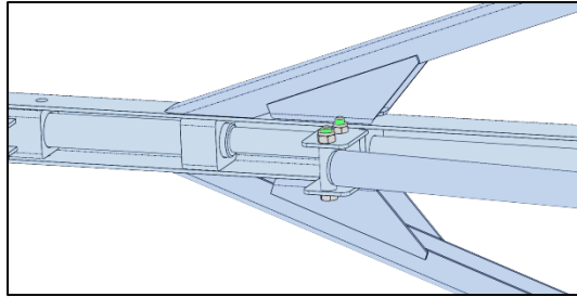
Druckgestänge der Auflaufeinrichtung – Anlage des Druckgestänges an der stirnseitigen Planfläche der Zugöse in Löseposition = Grundstellung
