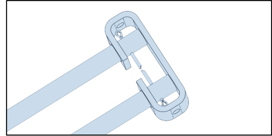
Höhenhalteeinrichtung der Zuggabel – bei korrektem Anbau müssen die Stützrohre in die dafür vorgesehenen Bohrungen eingeschoben und mit den beiden Splinten gesichert sein
