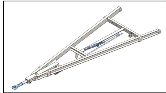
Zuggabel mit Auflaufeinrichtung – Fahrzeugtyp SWW560
