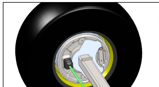
Einstellbolzen der Bremse des rechten Rades im Uhrzeigersinn drehen.
