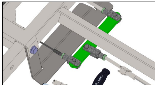
Bremszug wieder in Ausgleichswaage einbauen.
