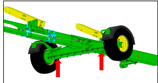
Wagenheber unter der Hinterachse positionieren und Hinterachse anheben.
