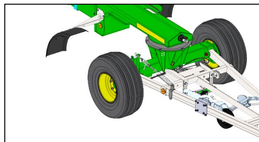
Linkes Rad in Fahrtrichtung nach vorn drehen.
