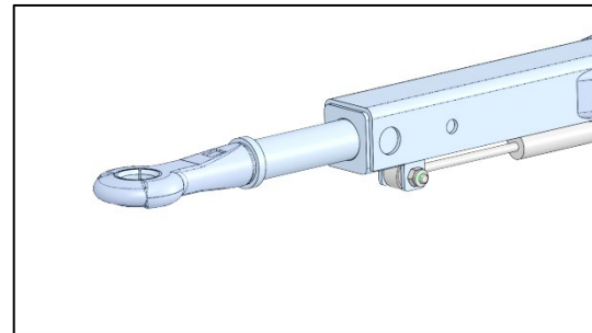
Auflaufeinrichtung – Zugöse in Löseposition = Grundstellung = ganz ausgefahren = 120 mm (SWW550) bzw. 140 mm (SWW500) möglicher Hub
