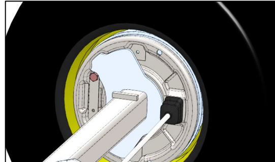
Einstellbolzen der Bremse des linken Rades im Uhrzeigersinn drehen
