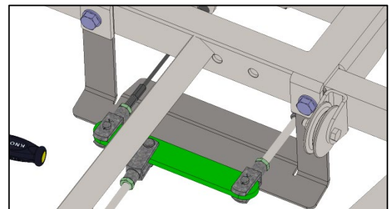
Zugstange der Zuggabel mit Ausgleichswaage verbinden.
