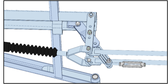
Druckgestänge der Auflaufeinrichtung – hinten in Führungsklotz eingeschoben; in Lösestellung des Druckgestänges = Grundstellung muss der Umlenkhebel nach vorn geneigt sein.
