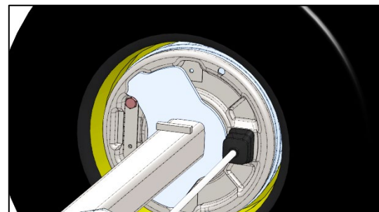
Einstellbolzen der Bremse des linken Rades im Uhrzeigersinn drehen
