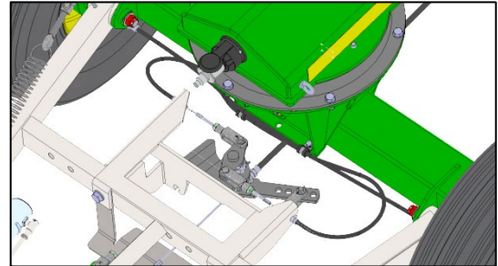
Bremszüge nach Einstellung der Bremsen der Vorderachse wieder in den Übersetzungshebel einbauen.
