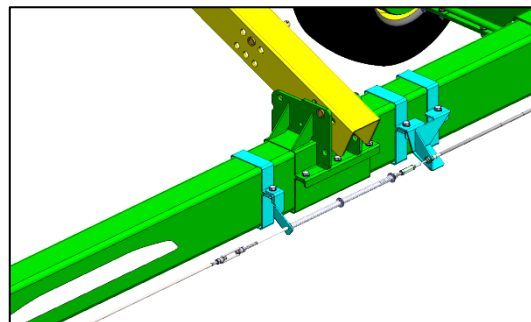
Einstellen der Radbremsen durch Drehen der Spannschloßmutter.
