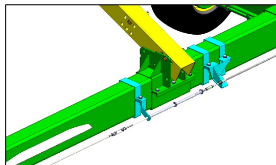
Einstellen der Radbremsen durch Drehen der Spannschloßmutter.
