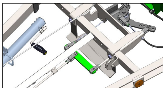
Verbinden des Seils der Übertragungseinrichtung mit der Spannschloßmutter der Auflaufeinrichtung.
