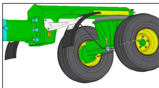
Nachstellschraube durch Drehen im Uhrzeigersinn anziehen.
