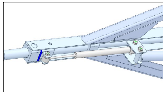
Hydraulischer Stoßdämpfer – in Löseposition = Grundstellung = ganz ausgefahren = 120 mm bzw. 140 mm Hub
