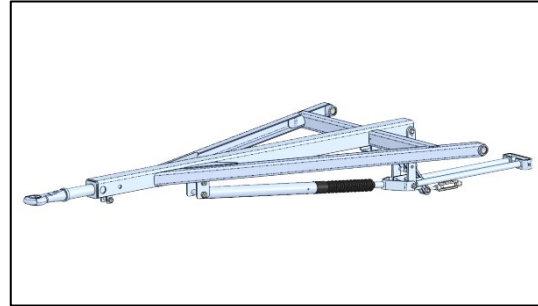
Zuggabel mit Auflaufeinrichtung – Fahrzeugtypen SWW500 und 550
