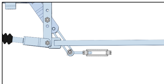
Auflaufeinrichtung – Umlenkhebel in Lösestellung = Grundstellung = nach vorne geneigt und am Druckgestänge anliegend; Kulisse nach hinten geneigt und Augenschraube mit Spannschloßmutter ganz nach hinten gezogen.
