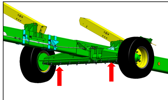
Unterstützung der Achse an den dafür vorgesehenen Punkten
