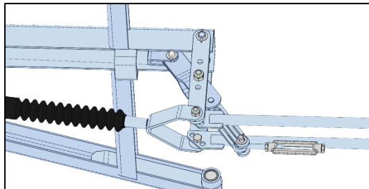
Höhenhalteeinrichtung der Zuggabel – bei korrektem Anbau müssen die beiden Verbindungshebel zwischen der Zuggabel und den Stützrohren bzw. der Höhenhalteeinrichtung („Klemmfix“) vertikal angeordnet sein.
